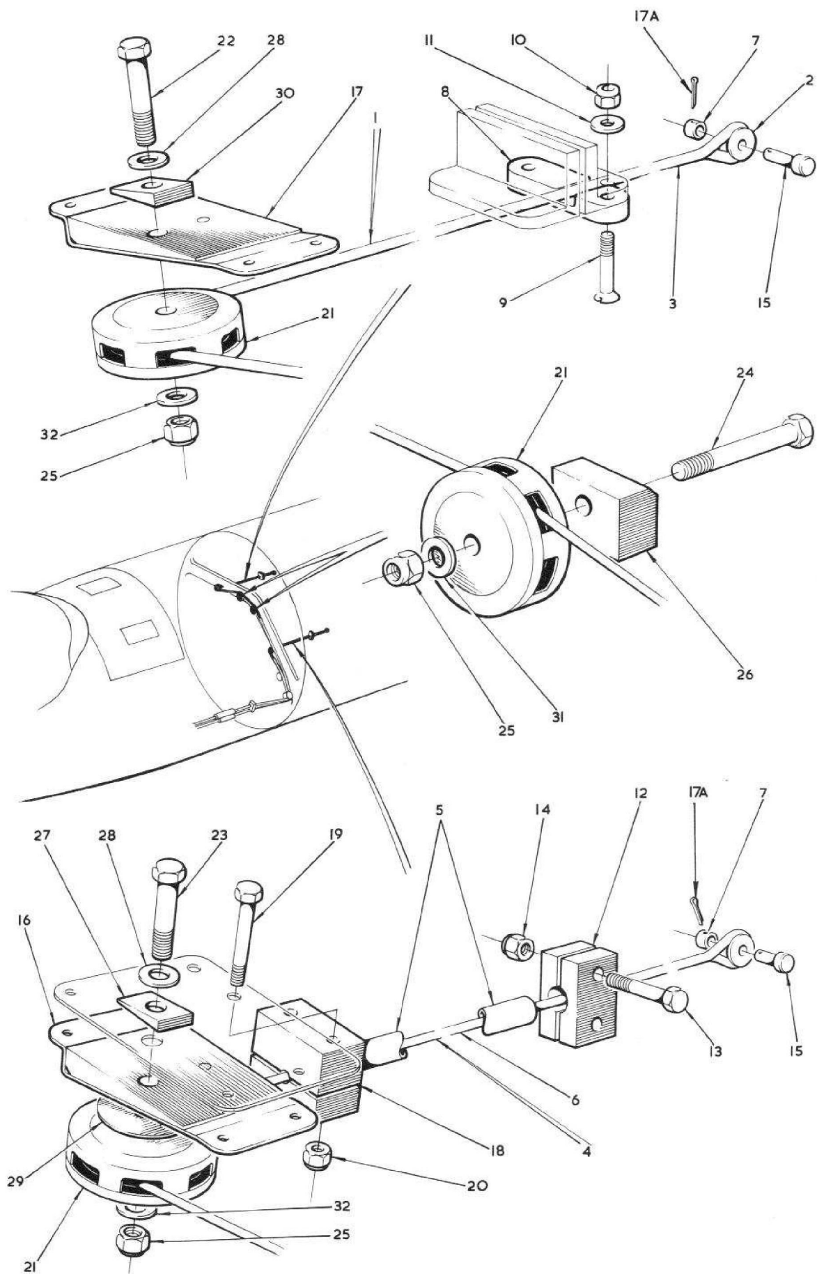
FIG. 2 CENTRE FUSELAGE
