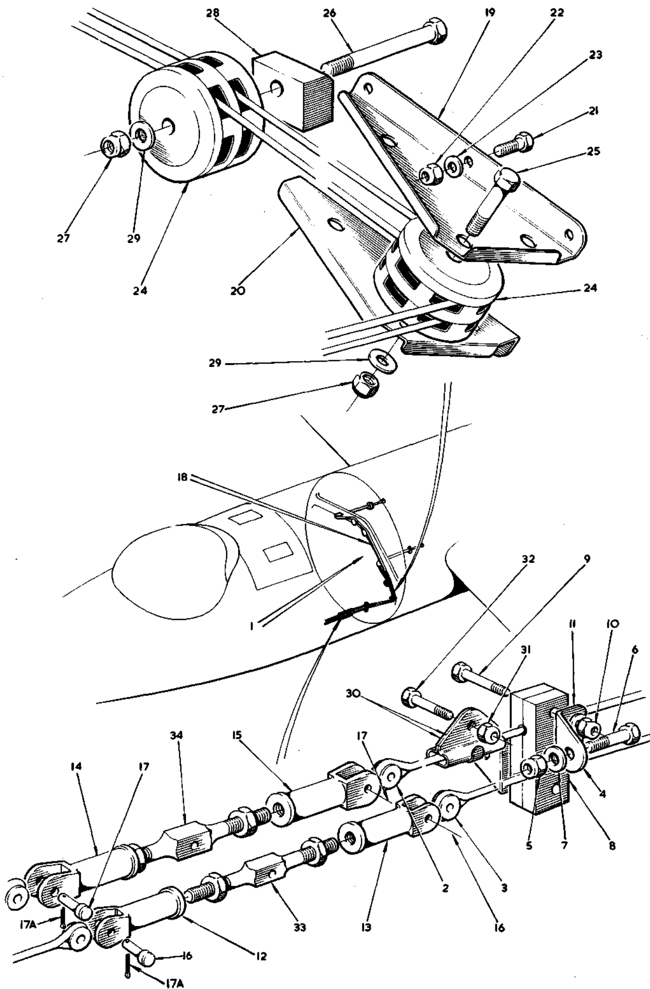
FIG. 1 CENTRE FUSELAGE
