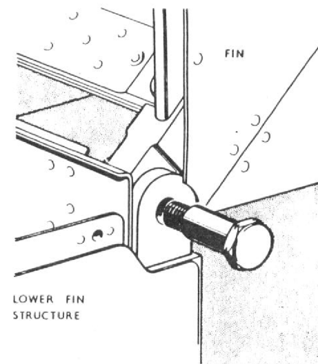
Fig. 7. Fin attachment—front
