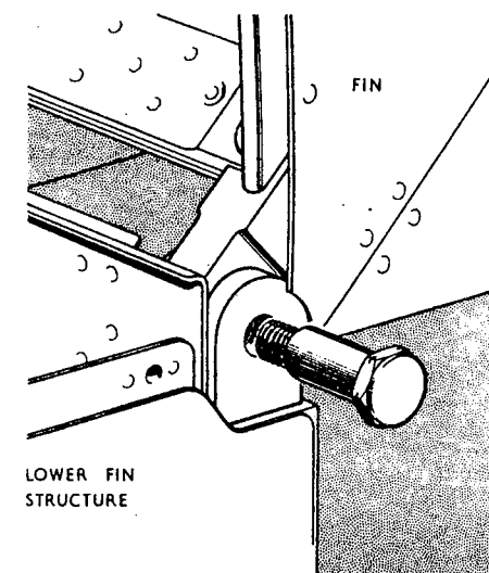
Fig. 7. Fin attachment—front
