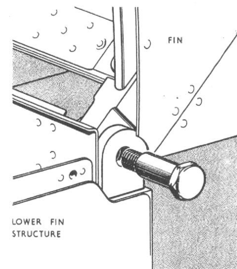
Fig. 7. Fin attachment—front
