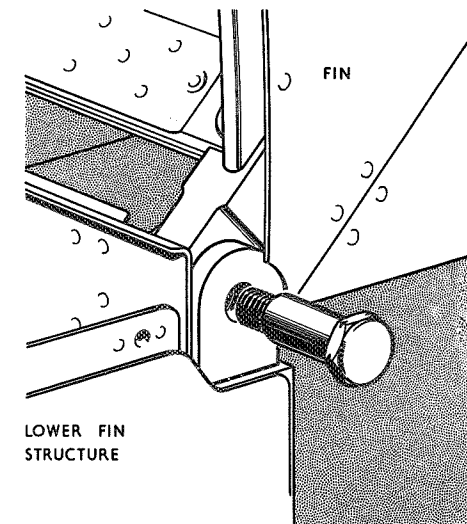
Fig. 7. Fin attachment—front
