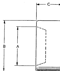
Fig. 39. Conduit ferrule Type G
