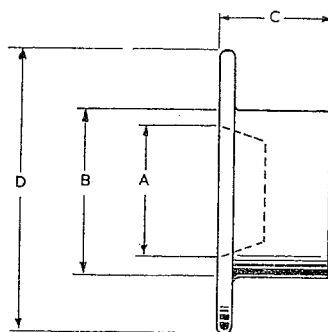
Fig. 38. Conduit ferrule Type H
