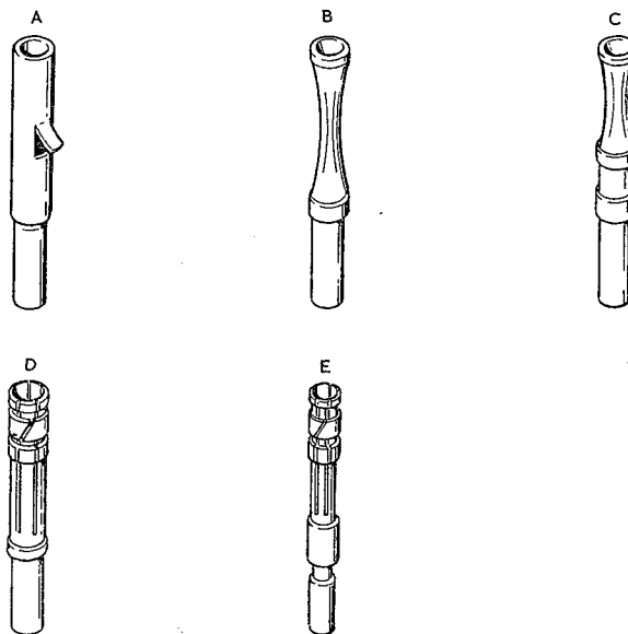
Fig. 21. Contacts
