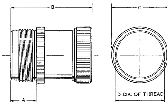
Fig. 28. Dimensions free unit
