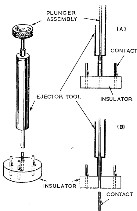
Fig. 19. Ejector tool
