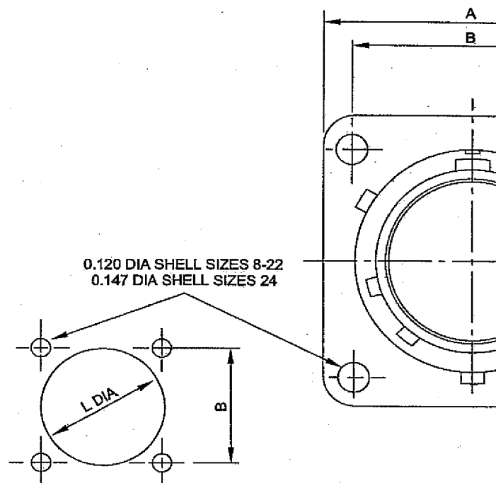
Fig 19 462H Square
