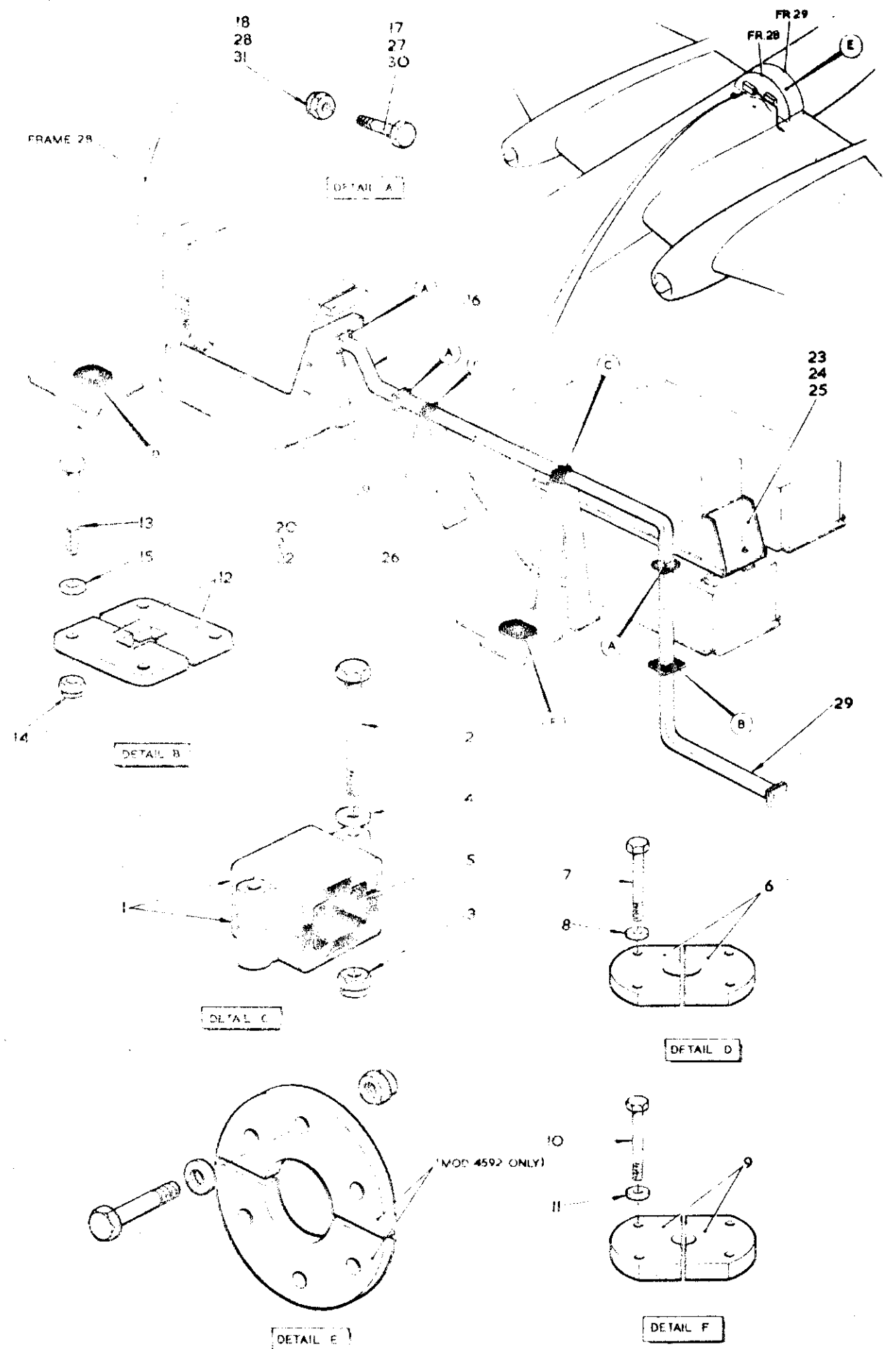
FIG. 2 DOPPLER NAVIGATOR
