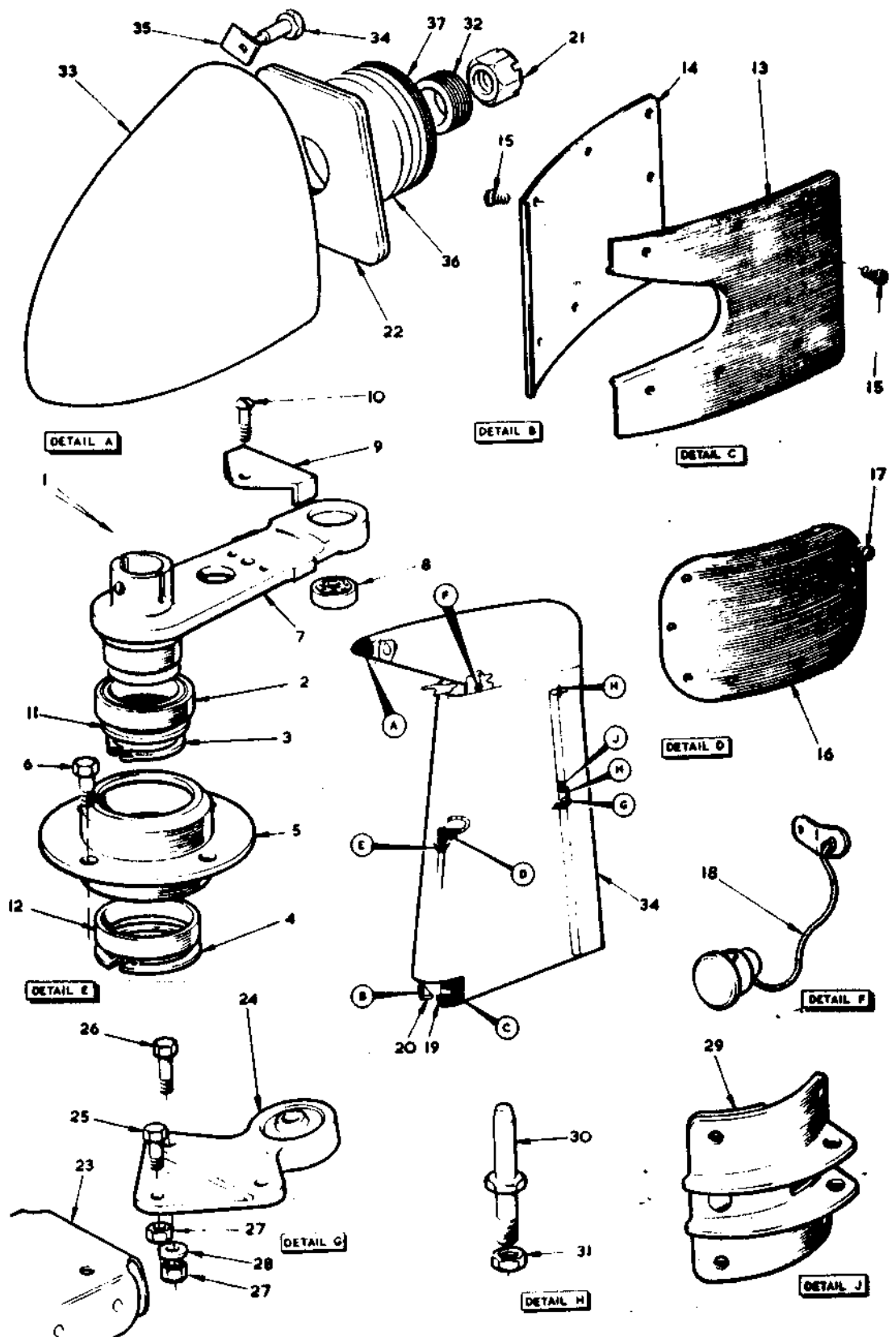
FIG. 3 RUDDER C/W TAB
