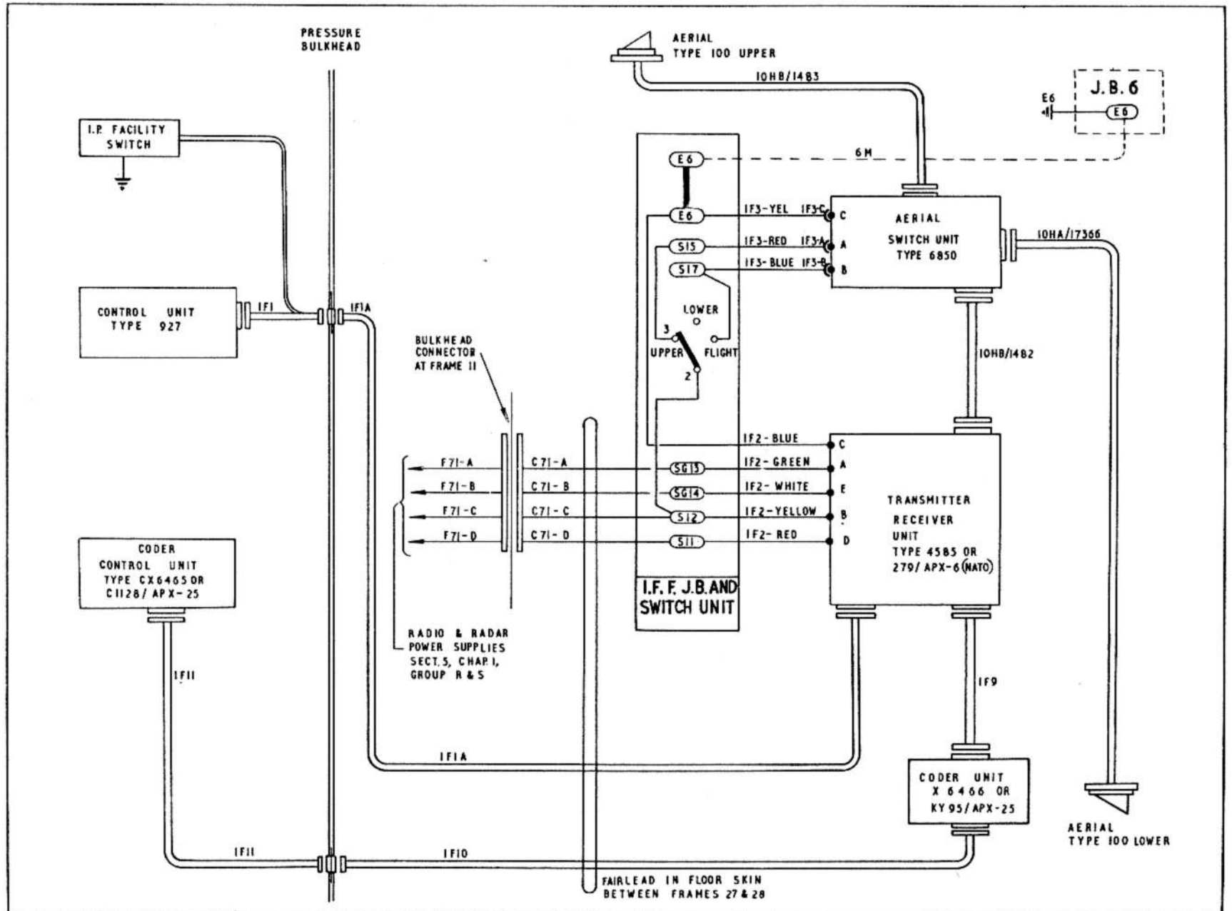
Fig. 3. I.F.F. Mk.10 (S.I.F.) - (A.R.I.5848)
