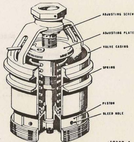
Fig.2. Spill valve
