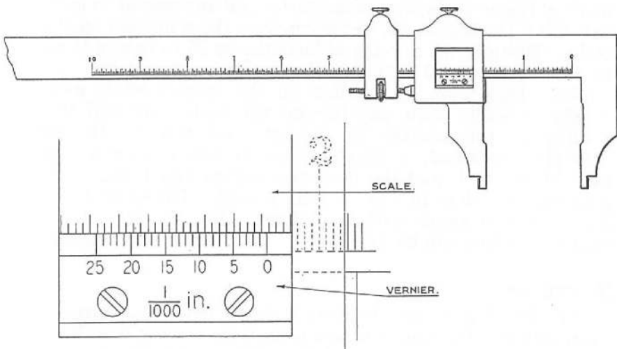
FIG. 7.—Vernier.
