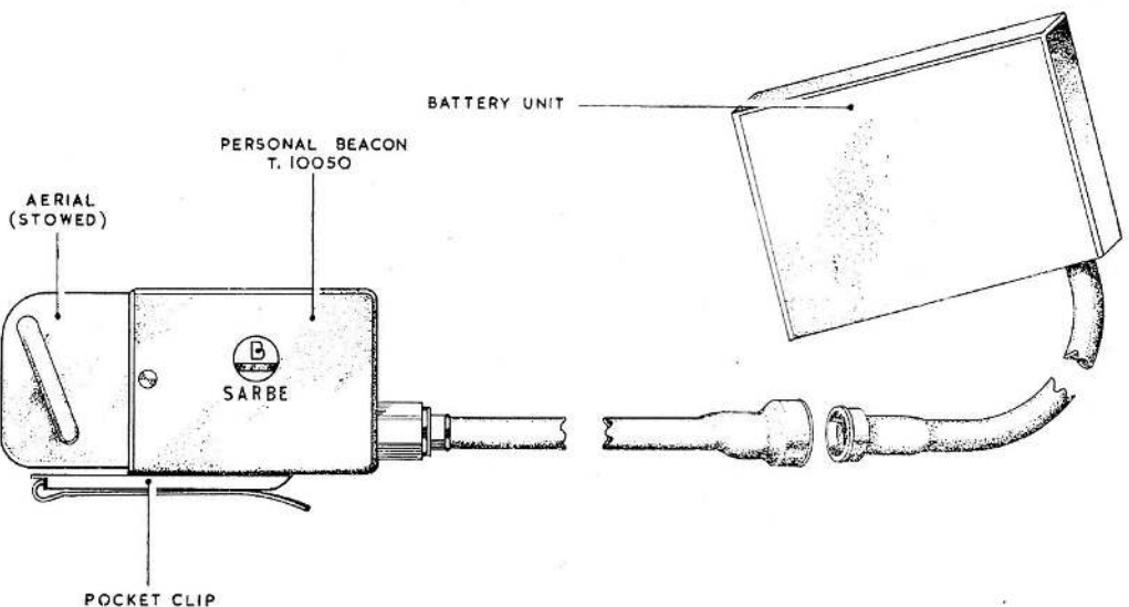
Fig. 3. Transmitter, Type T.10050 (S.A.R.B.E.)
