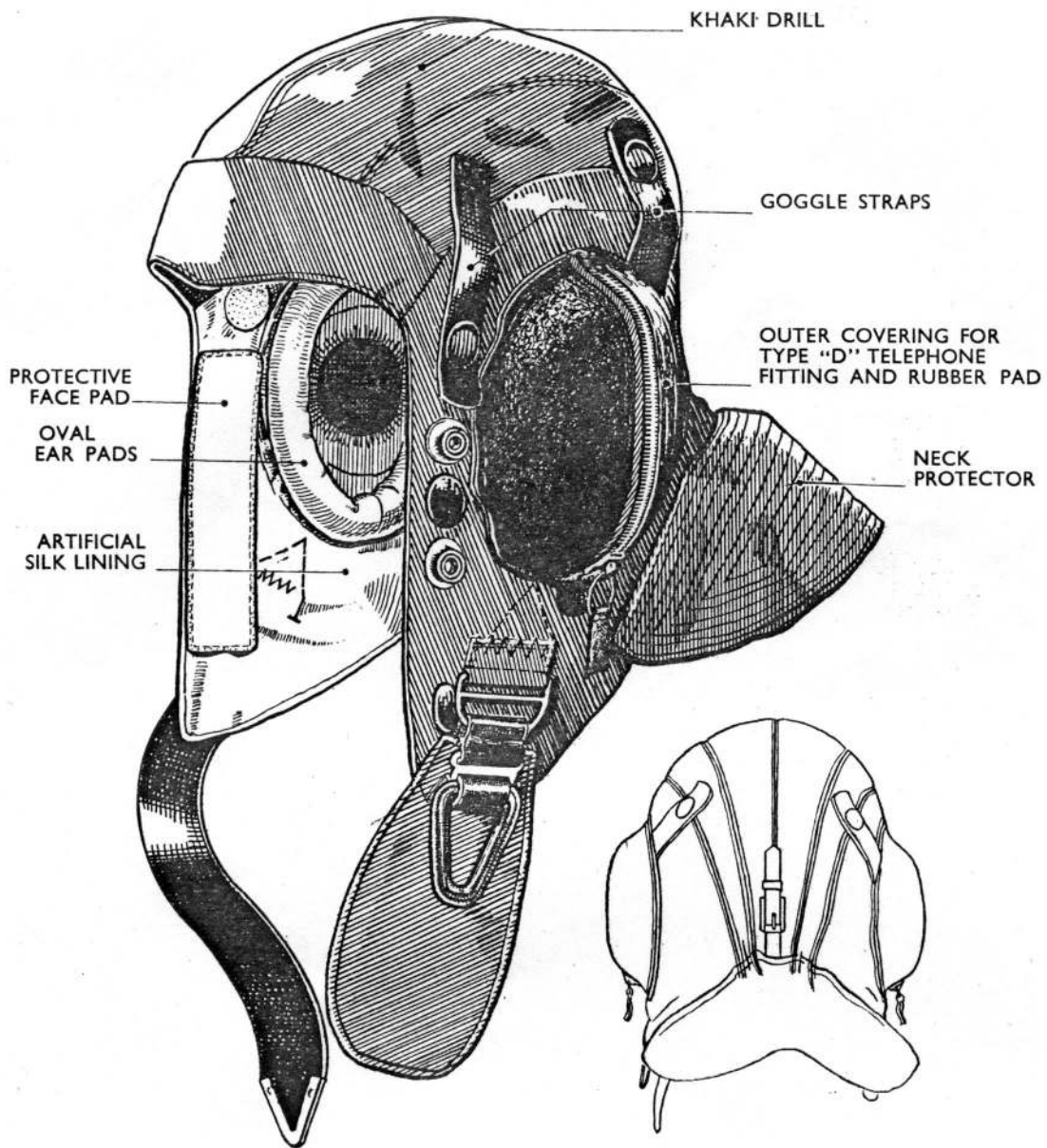
Fig. 7.—Naval helmet
