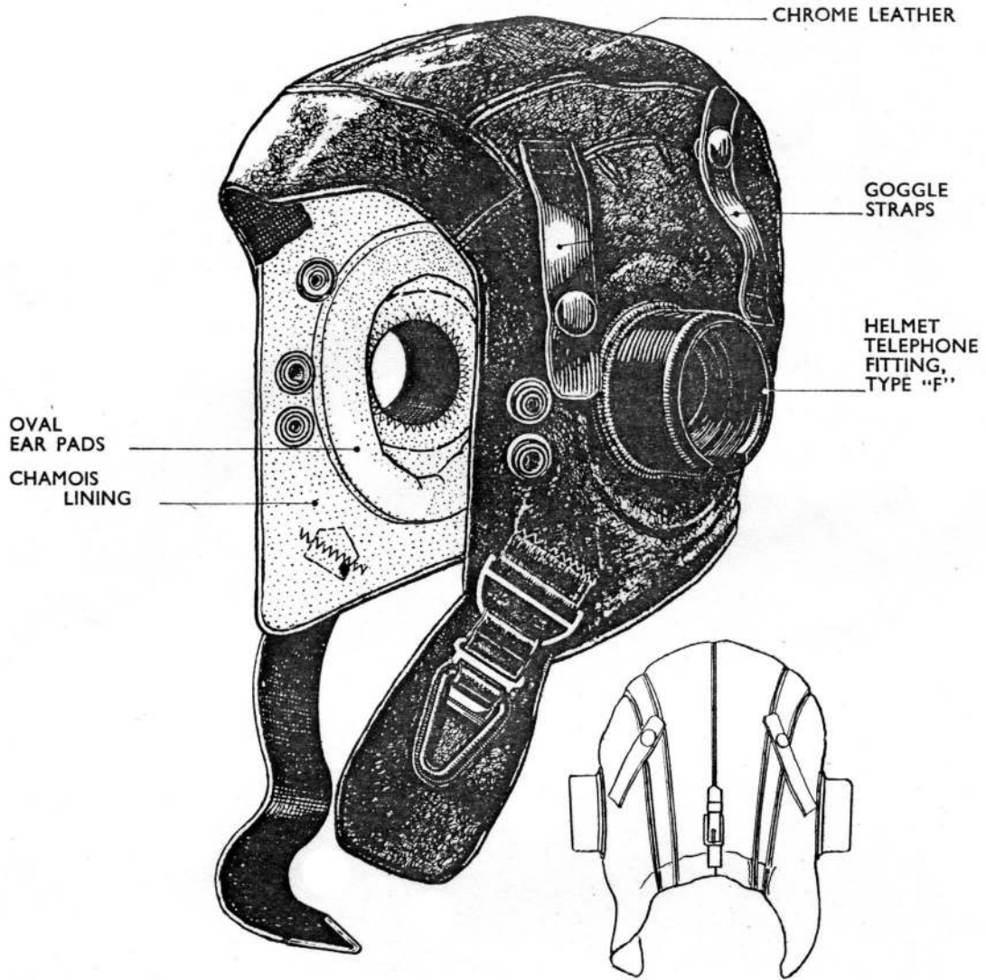
Fig. 1.—Type C helmet
