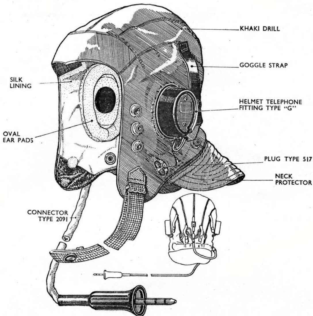
Fig. 5.—Type D wired helmet
