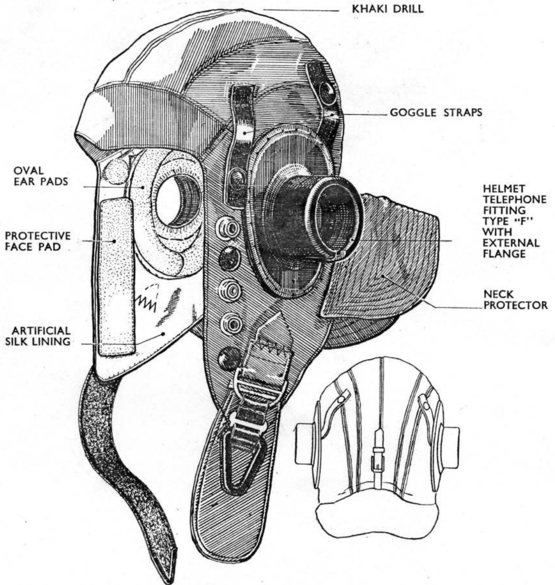
Fig. 2.—Type D helmet
