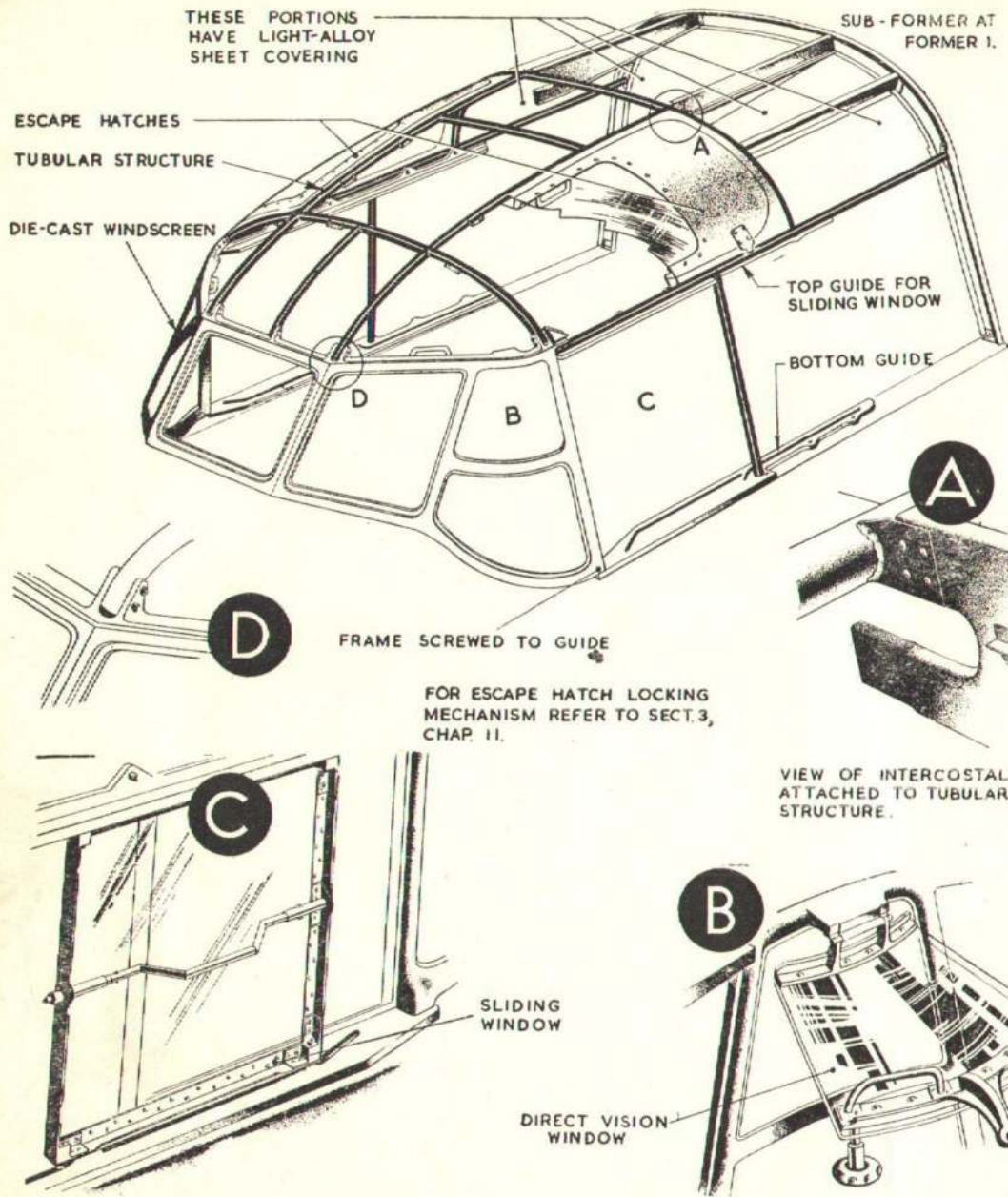
Fig. 11. Canopy
