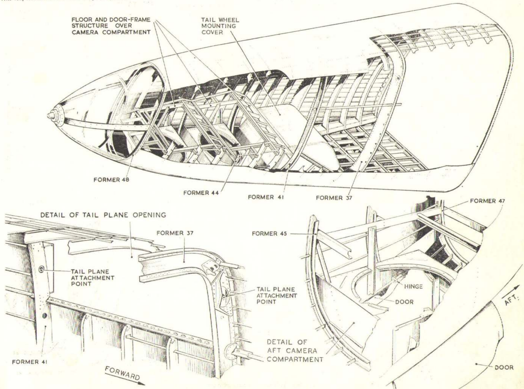
Fig. 20. Rear section
