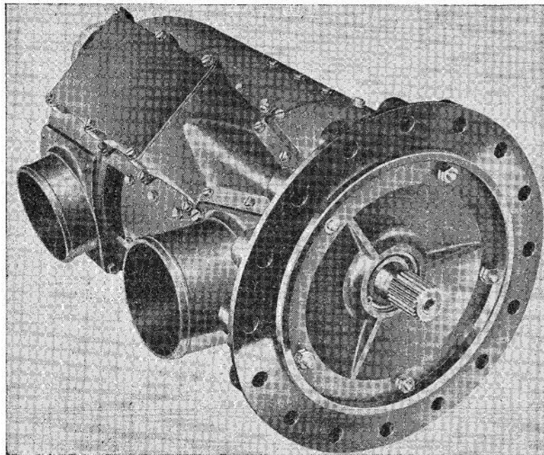
Fig. 1. Generator Type 512
