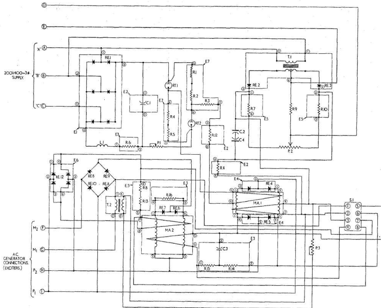
Fig. 5. Wiring diagram
