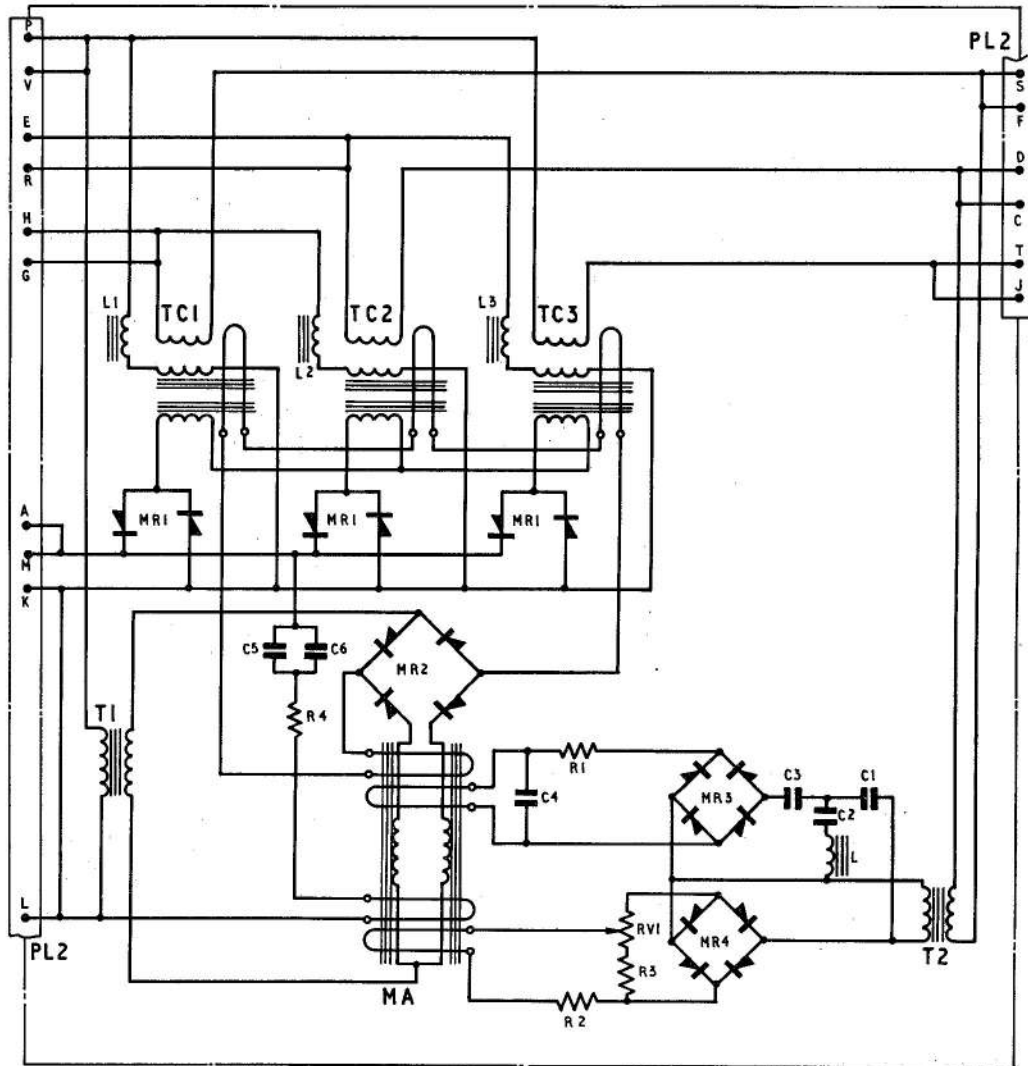
Fig. 2. Wiring diagram
