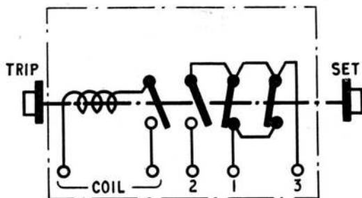
Fig. 3. Wiring diagram
