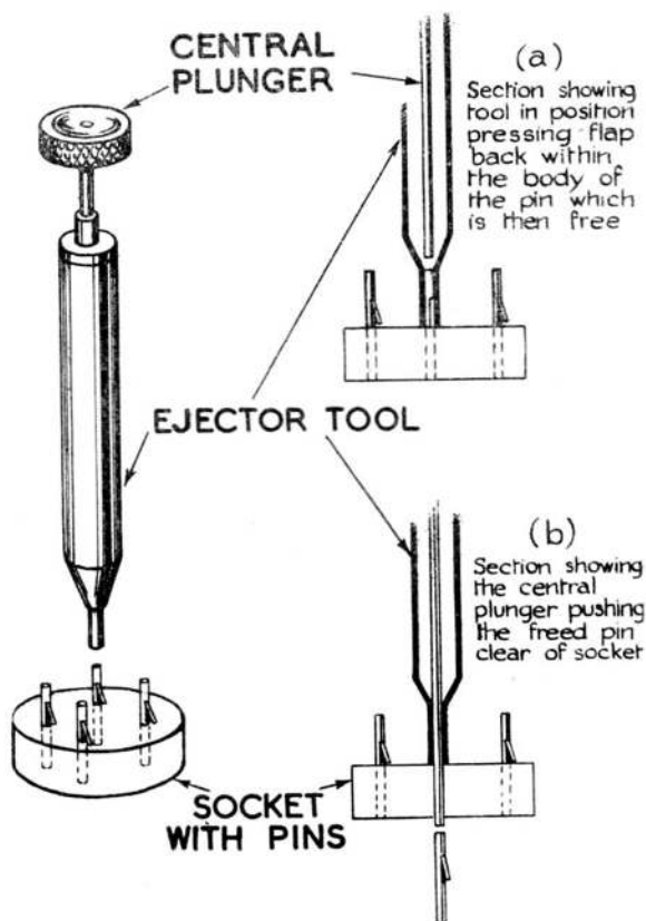
Fig. 19. Socket ejector
