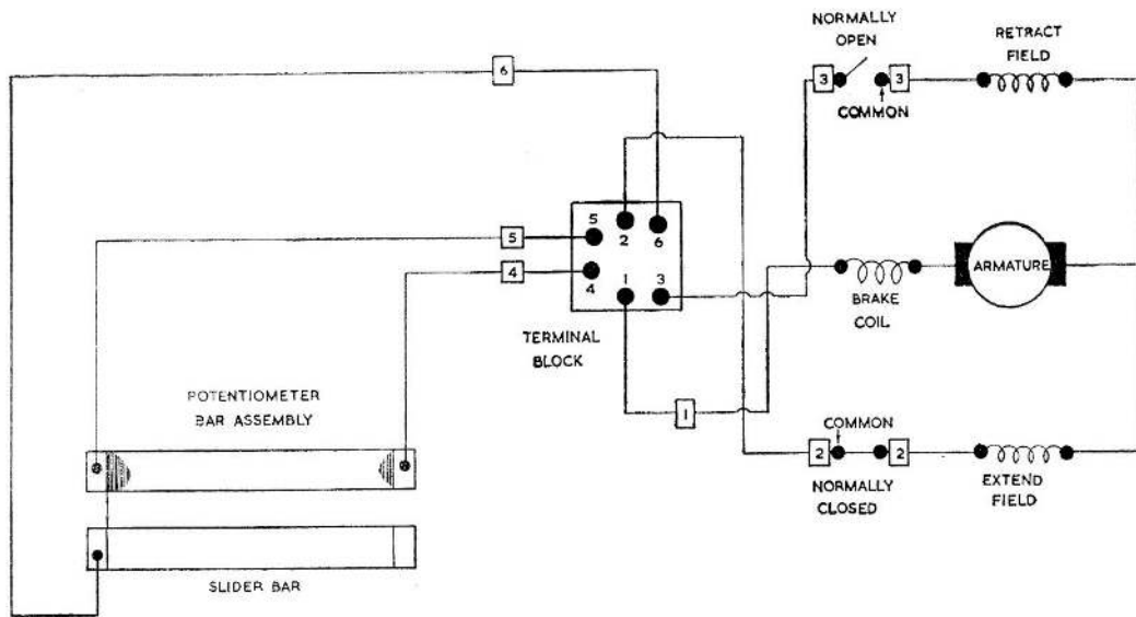
Fig. 4. Wiring diagram
