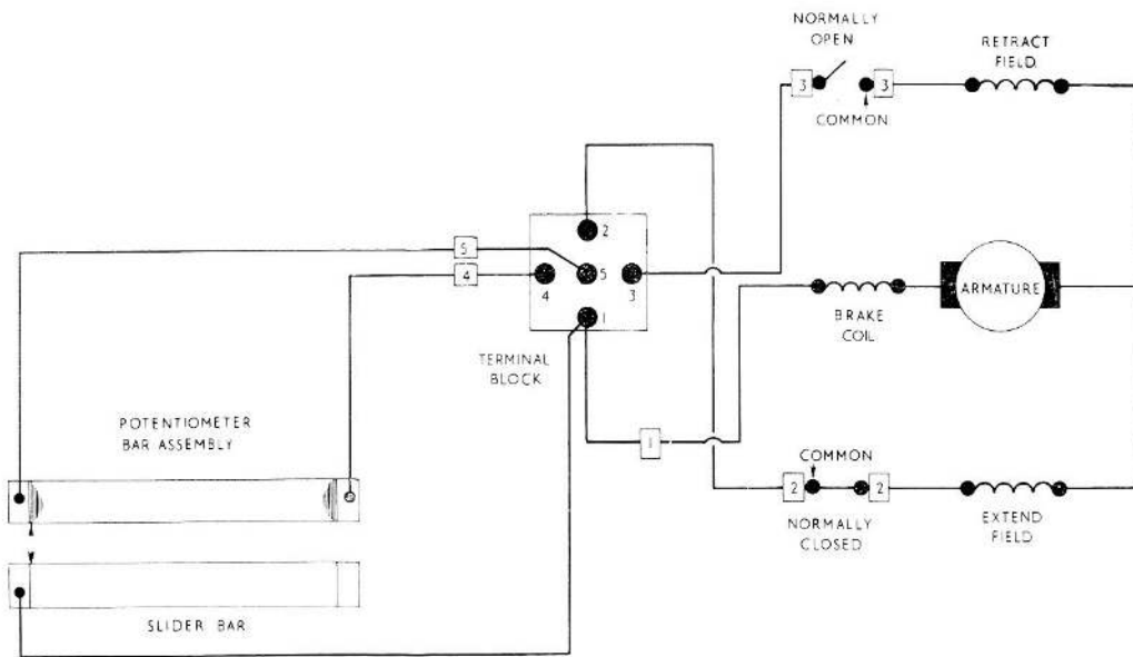
Fig. 2. Wiring diagram
