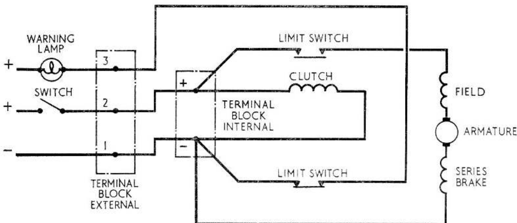
Fig. 4. Wiring diagram
