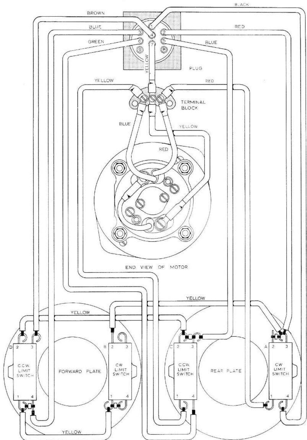
Fig. 5. Wiring diagram
