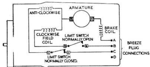
Fig. 4. Wiring diagram
