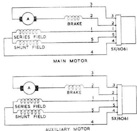
Fig. 2. Wiring diagram
