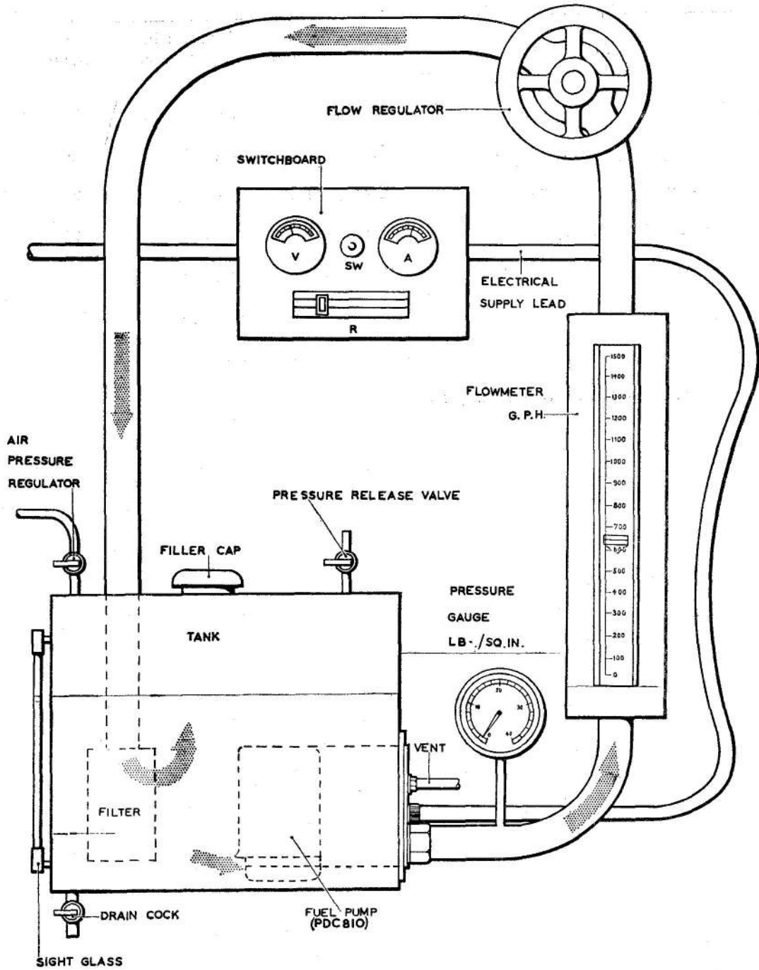
Fig. 9. Test rig
