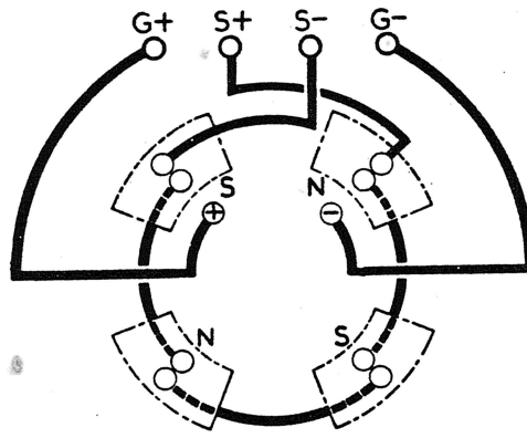
COUNTER-CLOCKWISE ROTATION
