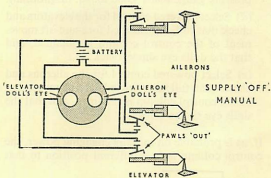
Fig. 16. Elevator Circuit
