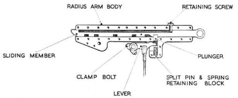
Fig. 7. Parachute container
