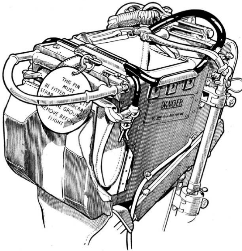
Fig. 8. Drogue container
