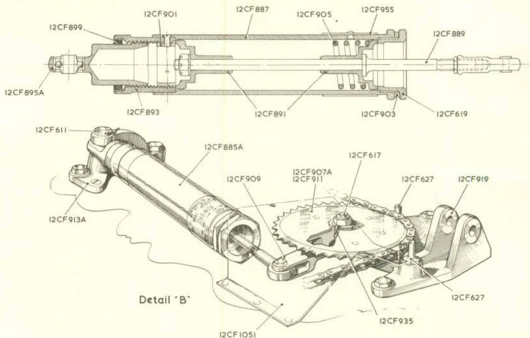
STRUT SPRING, AILERON.
