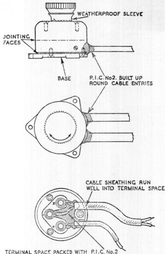
Fig. 4. Dimmer switch
