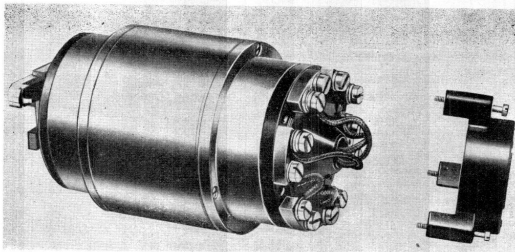
Fig. 12. Magslip hunter
