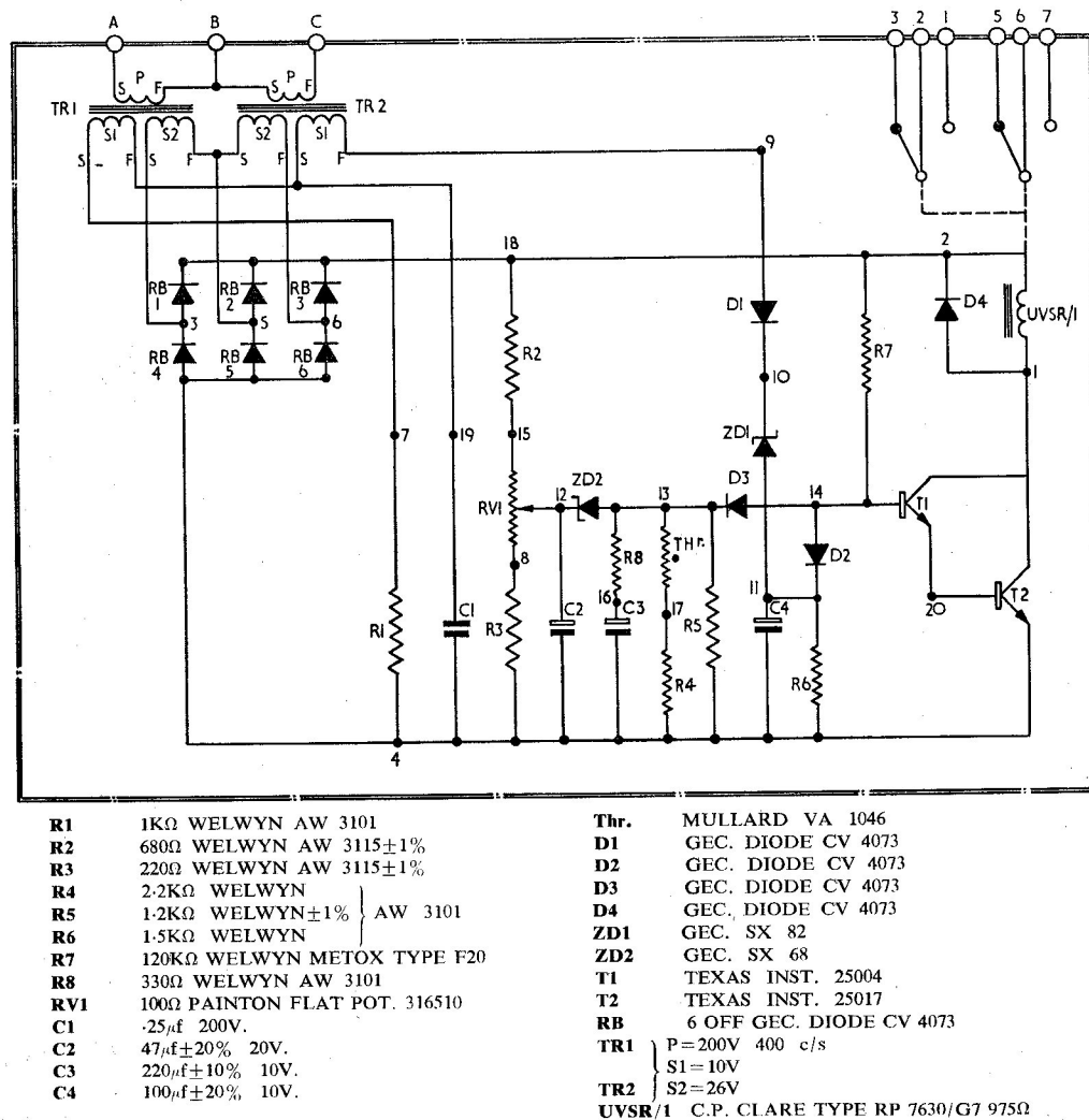
Fig. 3. Wiring diagram
