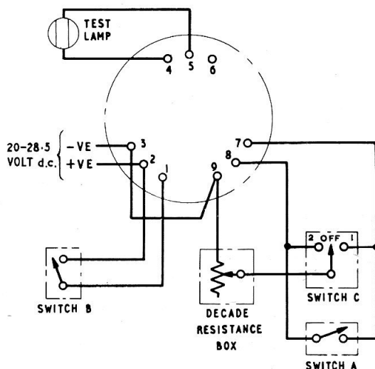
◀Fig. 1. Test circuit diagram▶
