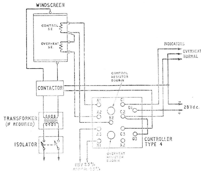
Fig. 7. Wiring diagram
