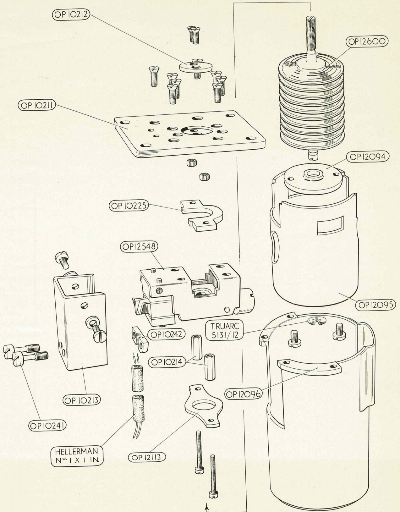
ALTITUDE SWITCH
